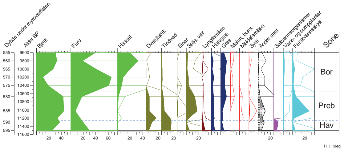
Figur 6. Pollendiagram over Gunnerødmyra som viser den eldste pionervegetasjonen og overgangen fra havbukt til et lite ferskvannstjern. De fiolette og lyseblå kurvene viser overgangen fra saltvanns- til ferskvannsmiljø (stiplet linje). I høyre side, sonene Bor: Boreal og Preb: Preboreal. Dette er en botanisk-geologisk inndeling av tiden etter istiden, også brukt som klimasoner.
