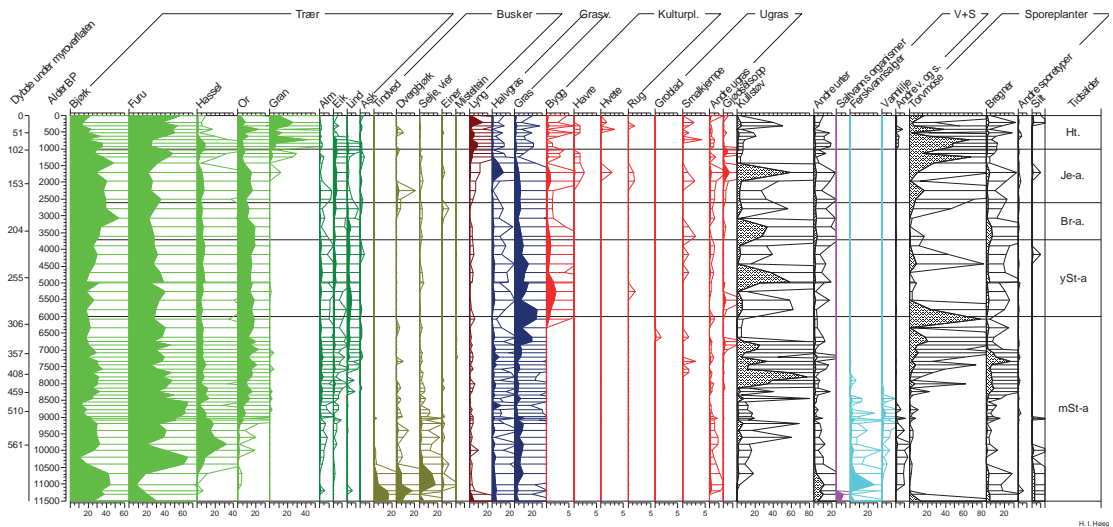
Figur 7. Utviklingen av vegetasjonen på og omkring Gunnerødmyra i de siste 11.500 år. Pollendiagrammet viser innvandringen av forskjellige trær, variasjoner i skogsbildet med busker, gras og blomsterplanter, bregner og torvmoser gjennom 11.500 år. V + S: Vann- og sump-planter. Kurven for kullstøv kan si noe om åkerrydding i skogen, men det kan også ha vært skogbranner. Mer forklaring av pollendiagrammet, se faktaboks.
