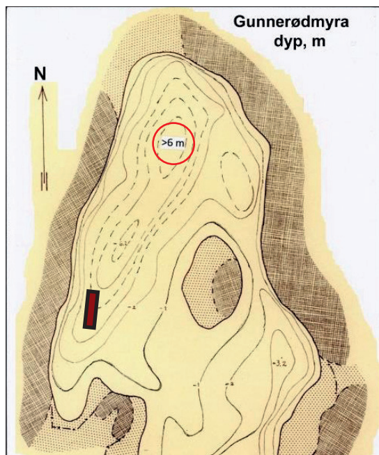
Figur 2. Dybdemålinger i nordre del av Gunnerødmyra. 1 m mellom linjene. Skraverte felt: Grunnlent med «skjæljastein», eller bart fjell i overflaten. Prikker: Sandjord.
