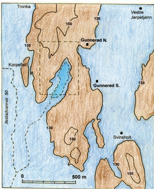
Figur 5. For omtrent 11.200 år siden var havnivået 130 m høyere enn i dag. Da var utbredelsen av hav og land slik som vist på figuren.
